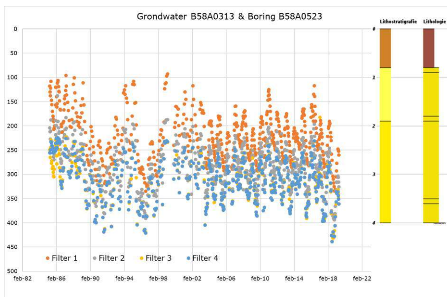
Figuur 3.6: Boven: De grondwaterstand- en stijghoogtefluctuaties t.o.v. maaiveld in meetpunt B58A0313. Filterdieptes t.o.v. maaiveld (+30.35 m NAP): filter 1 ca. 3 m, filter 2 ca. 8 m, filter 3 ca. 16 m en filter 4 ca. 23 m. Onder: de fluctuatie van de freatische grondwaterstand t.o.v. NAP (blauwe horizontale lijn is lokaal streefwaterpeil, de rode gearceerde lijn is 30 cm -mv).
