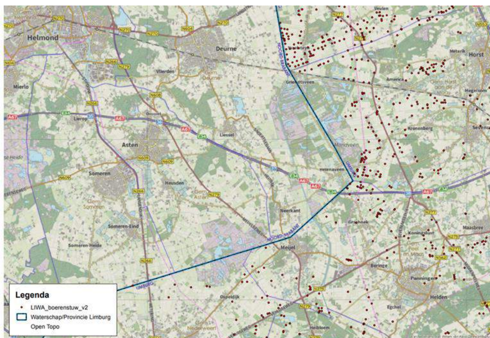
Figuur 2.5: Ligging boerenstuw_tjes LIWA model (alleen aan de Limburgse zijde van de Peelvenen).
