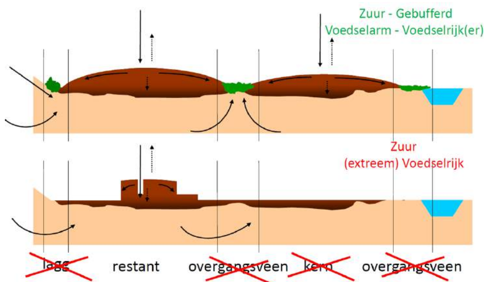
Figuur 4.4: Schematische weergave van een hoogveenlandschap (boven) en de situatie (onder) die meer representatief is voor de huidige toestand van de Peelvenen (Van Duinen, 2013).
